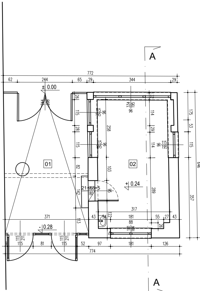
RZUT PRZYZIEMIA
