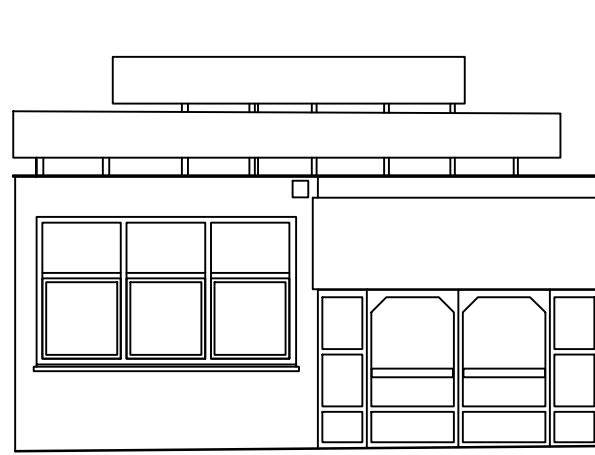
ELEWACJA ZACHODNIA
