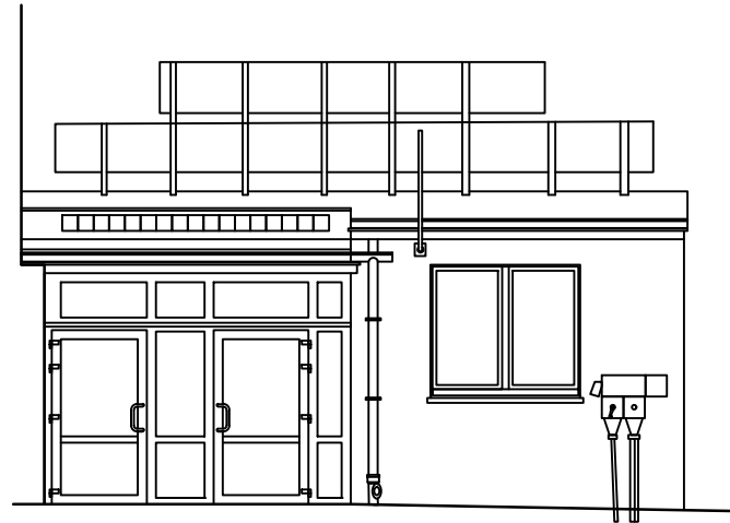
ELEWACJA WSCHODNIA
