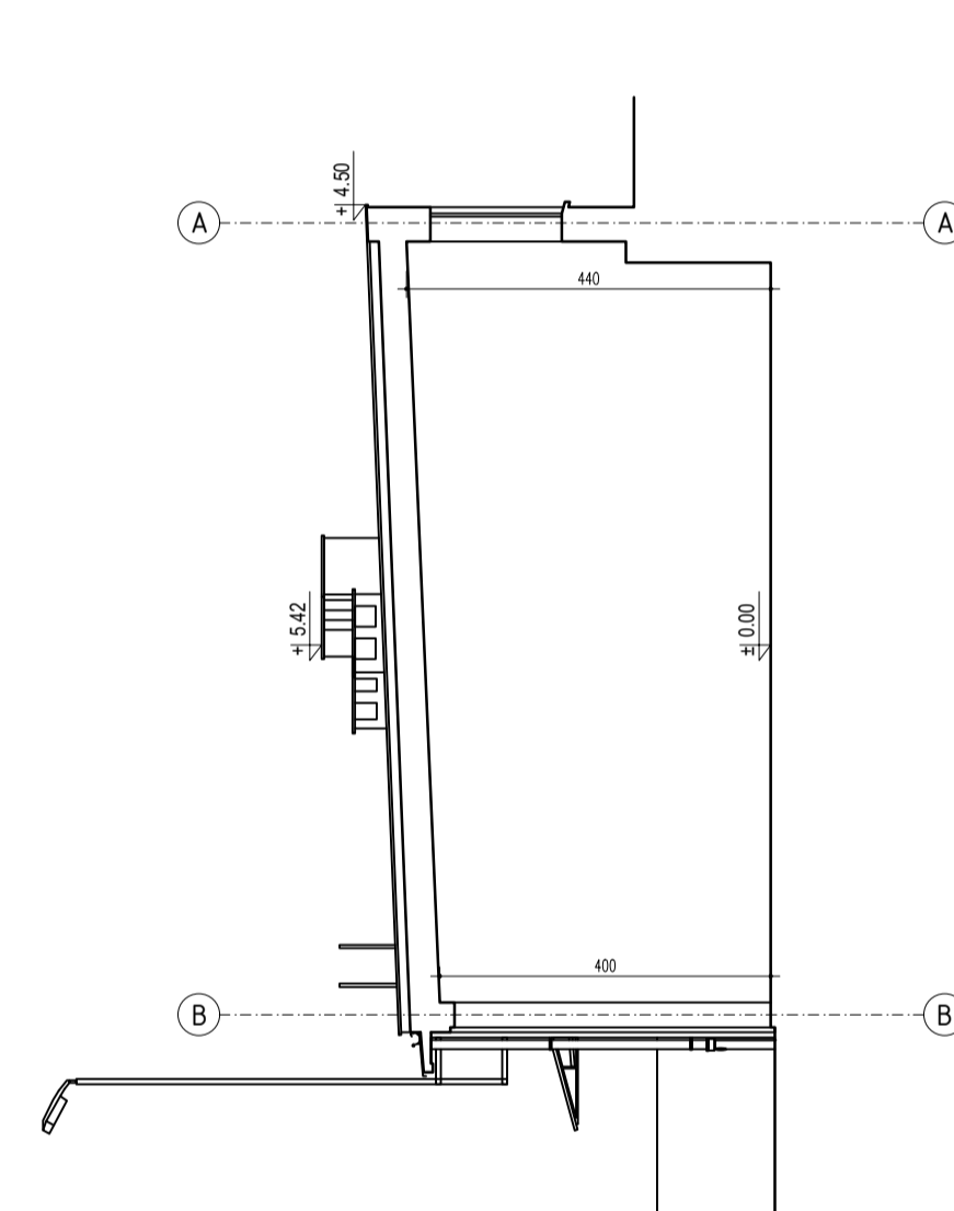
PRZEKRÓJ A-A
